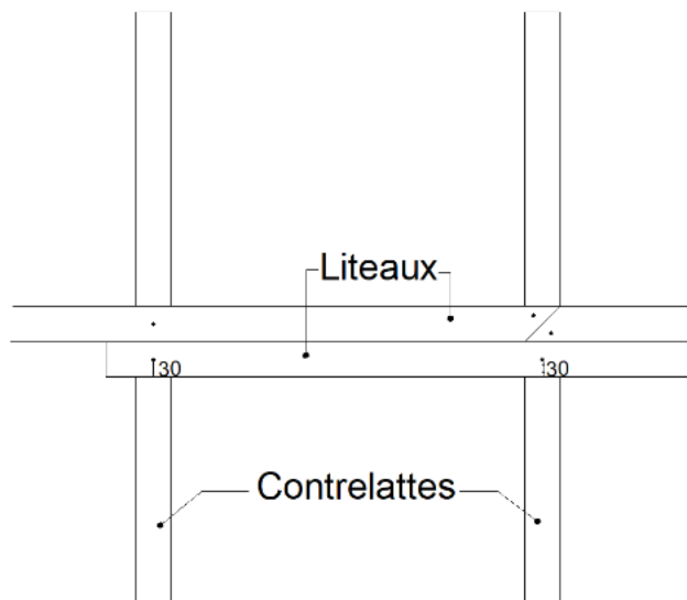
Figure 12 - Distance minimale à respecter pour la fixation du liteau sur la contrelatte : à gauche en partie courante, à droite lorsque les liteaux sont raboutés.
