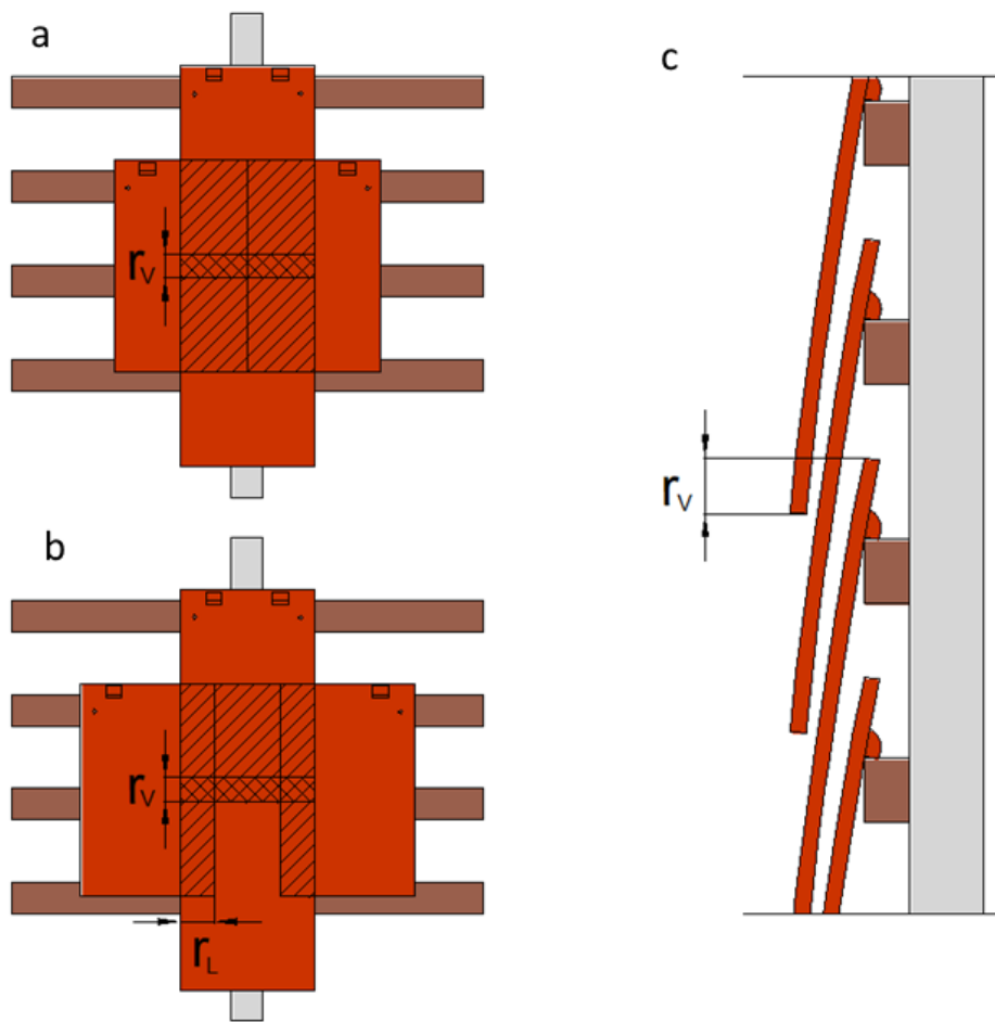
Figure 15 – a) Recouvrements minimaux à respecter en pose jointive. b) Recouvrements minimaux à respecter en pose jointive à claire-voie. c) Recouvrement transversal minimal.
