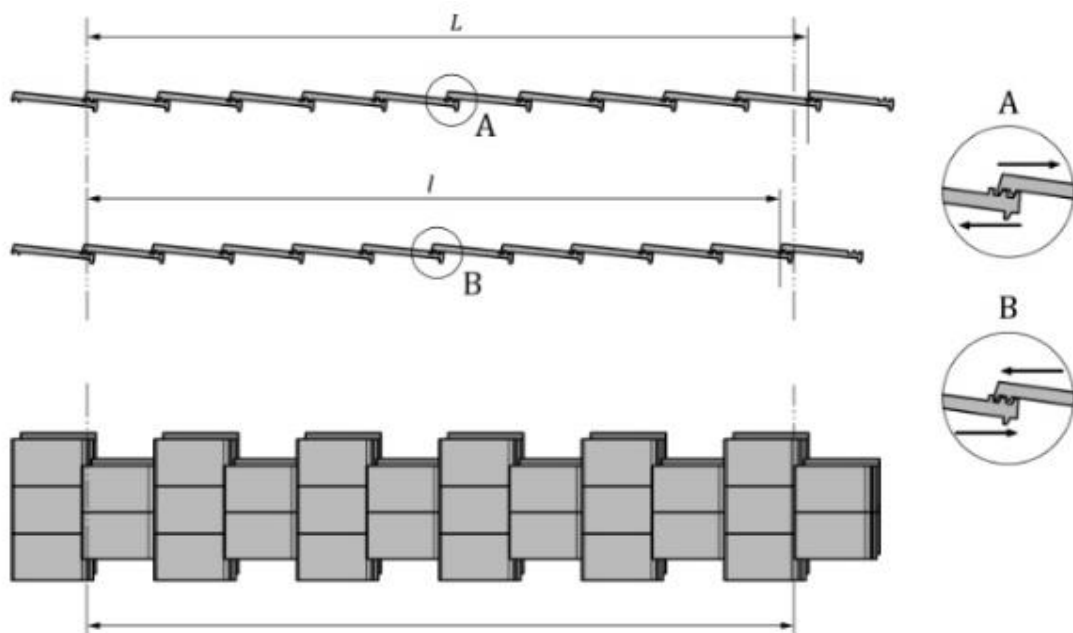
Figure 19 : schéma explicatif de la détermination du pureau pour les tuiles à emboîtement
